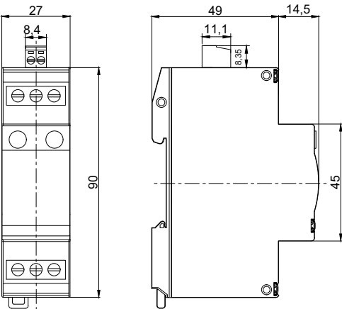
Габаритные размеры
